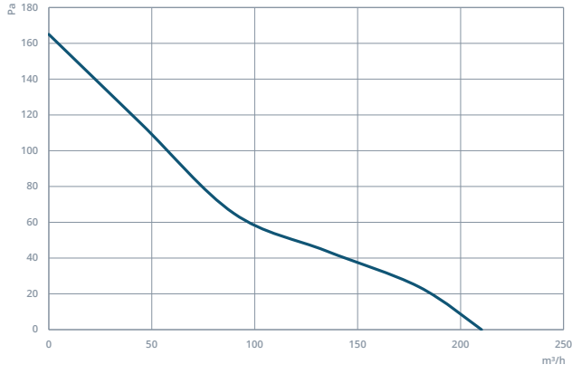
KAP 100
