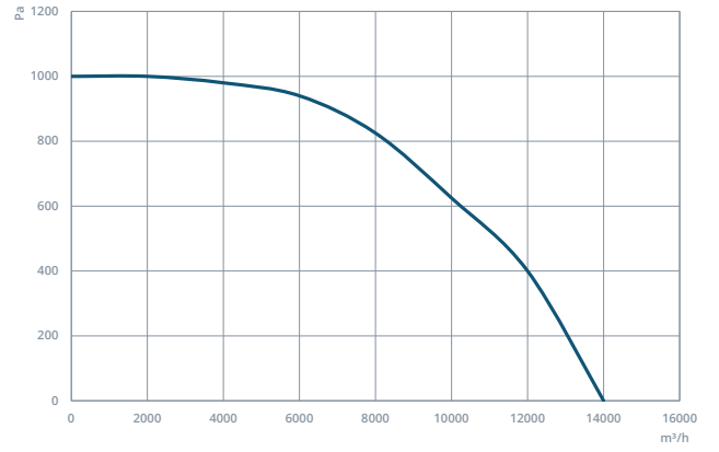
HMEF 630
