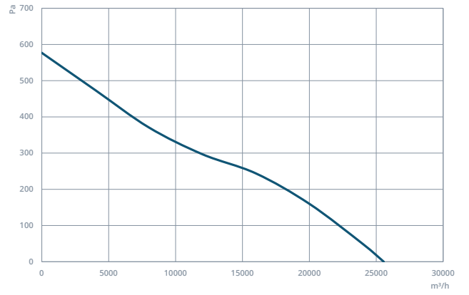
PAXI 800-5-30
