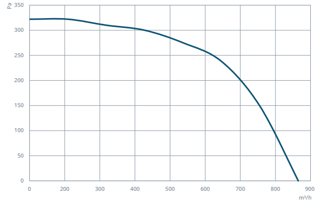
EC-RAD 160
