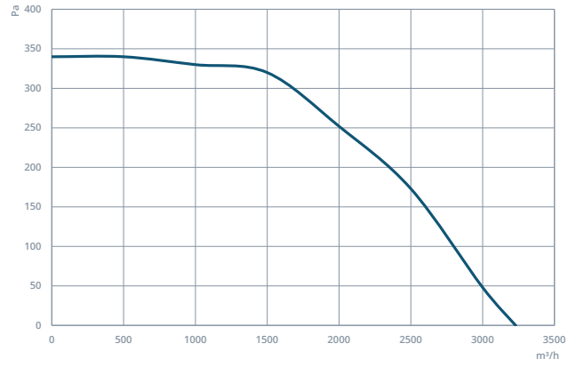
FFU 30
