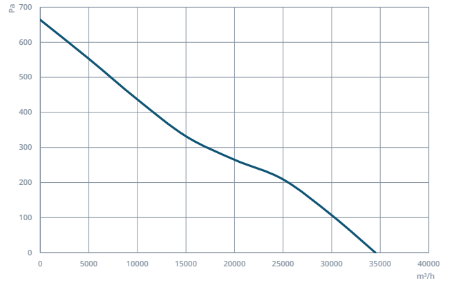
BAXI 900-5-35
