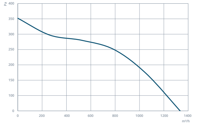
KAP 250
