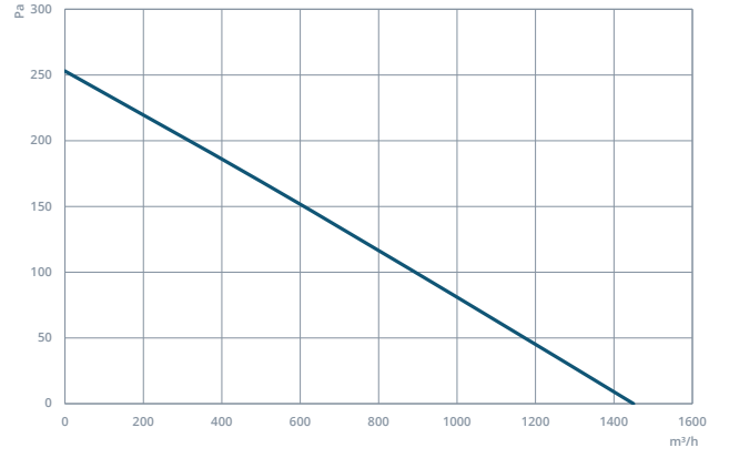
CAXIDIK 450-5-25
