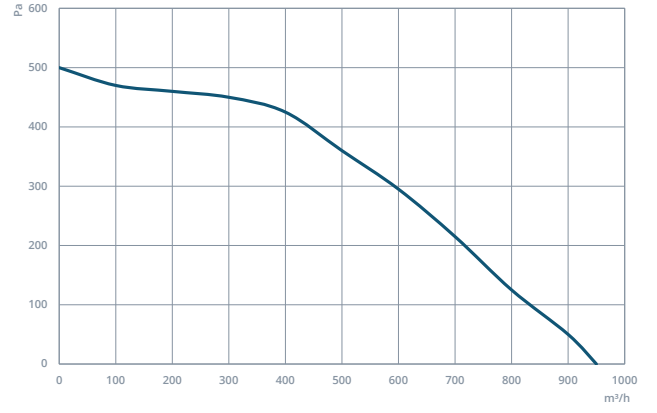
REC 40-20A
