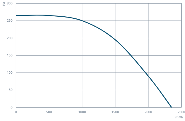
CRADIK 355
