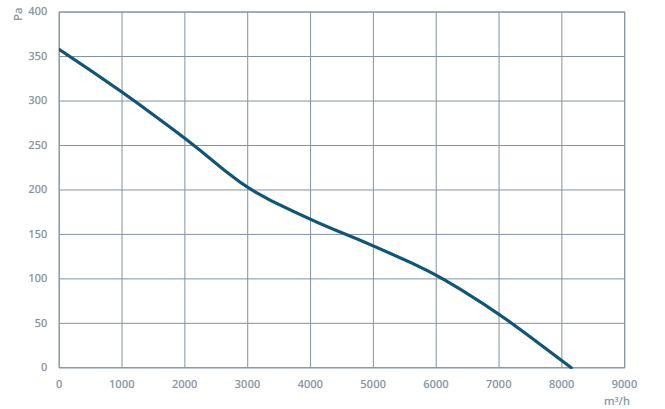
AXIP 560-5-25
