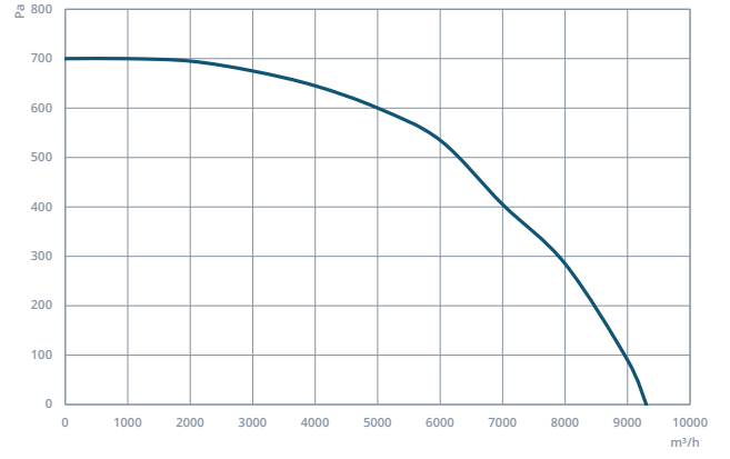
REC 100-50
