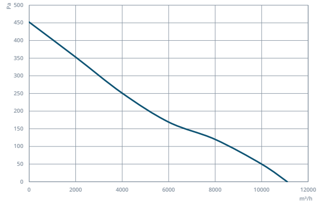
CTAXI 630-5-30
